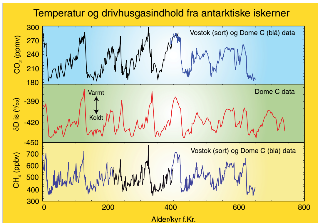
Data fra to antarktiske iskerner, der viser CO 2 -koncentrationen, δ-Deuterium (der er et indirekte mål for temperatur) og CH 4 -koncentrationen gennem de seneste 650.000 år. De tre parametre svinger stort set i takt og antyder, hvordan drivhusgasserne fungerer som en del af feedback-systemet, der forstærker temperaturændringer. (Grafik: UVH modificeret efter www.pages.unibe.ch )
